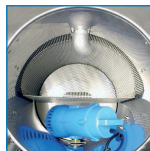
Pompe intégrée et tamis grossier
